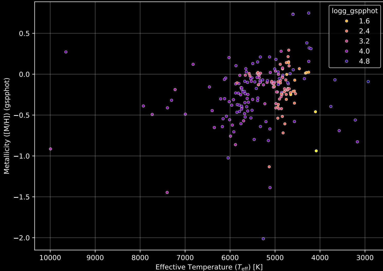
APOGEE DR17 Field: [182+30_MGA] Stellar Population Parameters (n= 200)
